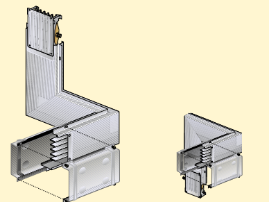
DX + DX (Тип 1)
